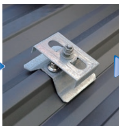
金具の台座を横位置に回し
