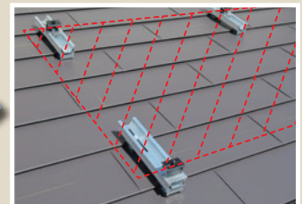
③押え金具でソーラーパネルを固定し、付属ナット (M8) で留付けます。
