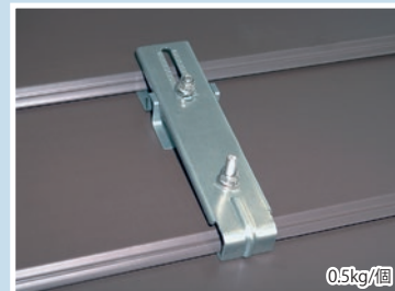
▲ダンビー 190用(ラック工法)
