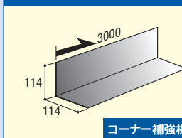
コーナー補強板 L
