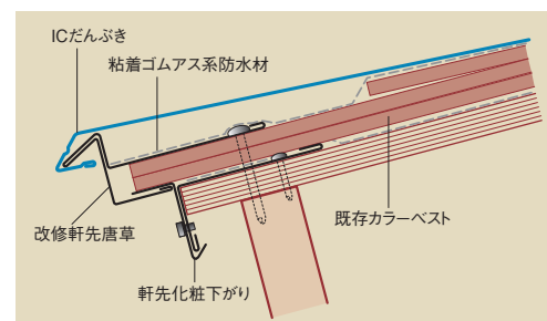
軒先部納め例
