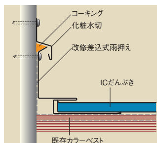
雨押え部納め例
