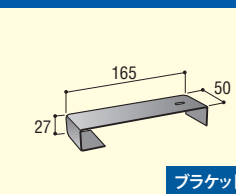
ブラケット C
