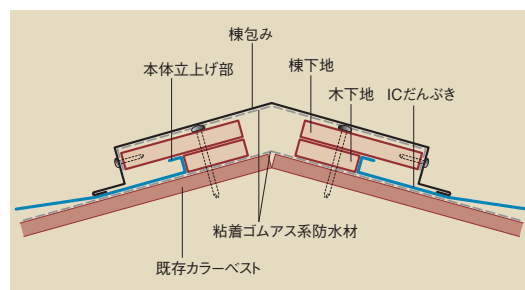
棟部納め例
