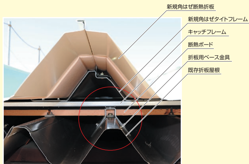
改修した断熱二重葺きの断面
