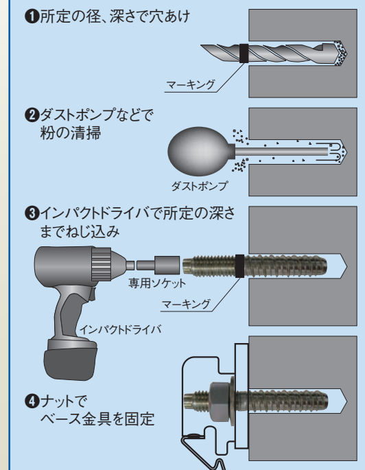
RC用タップスター
